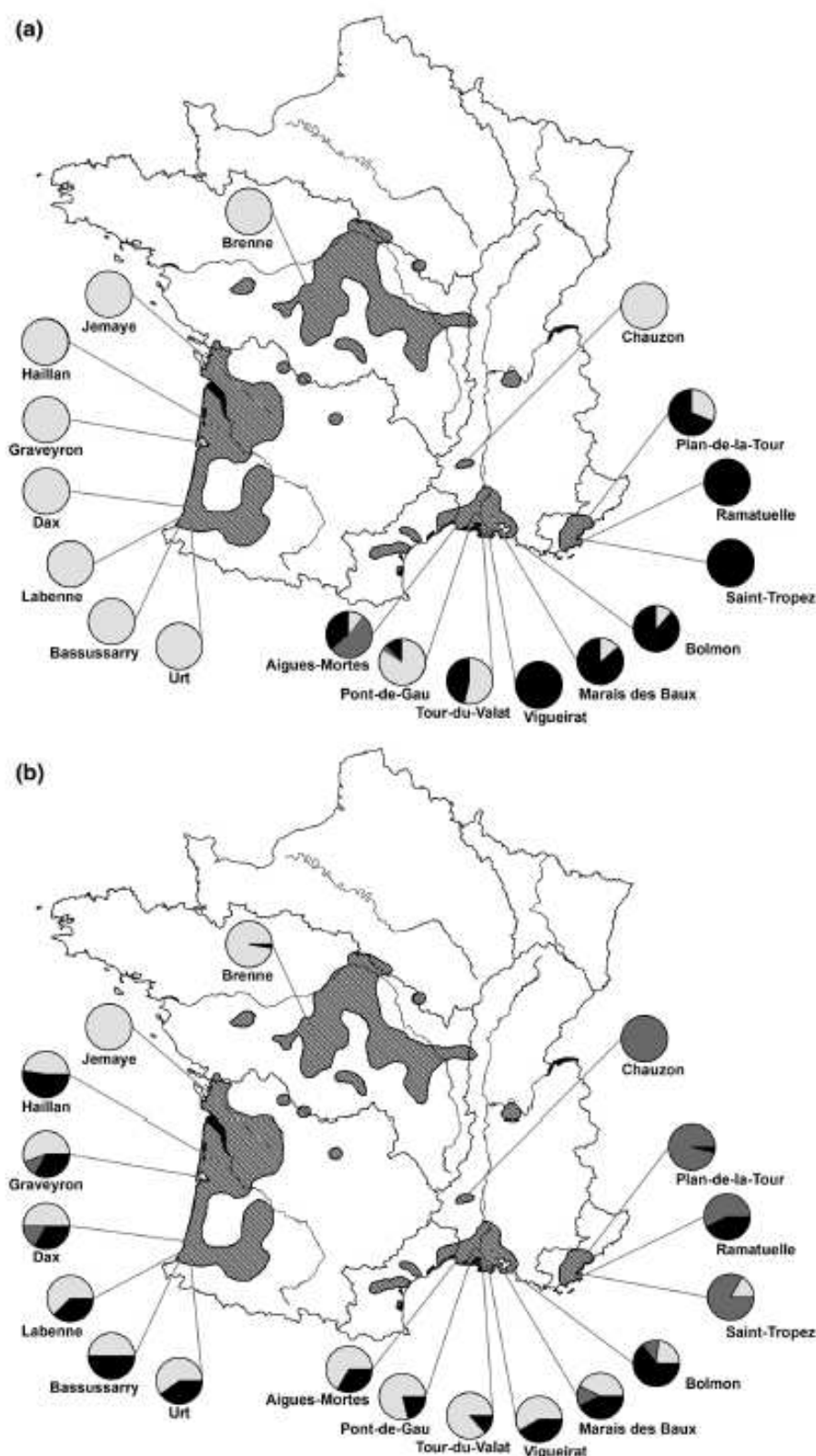
Figure 12 - Étendue géographique de la zone de contact entre les sous-espèces d' Emys orbicularis en France et niveaux d'introgression dans chaque population (Raemy et al., 2016).
