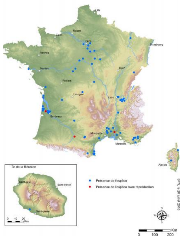
Figure 19. Distribution de la Tortue serpentine en France métropolitaine et en outre-mer
