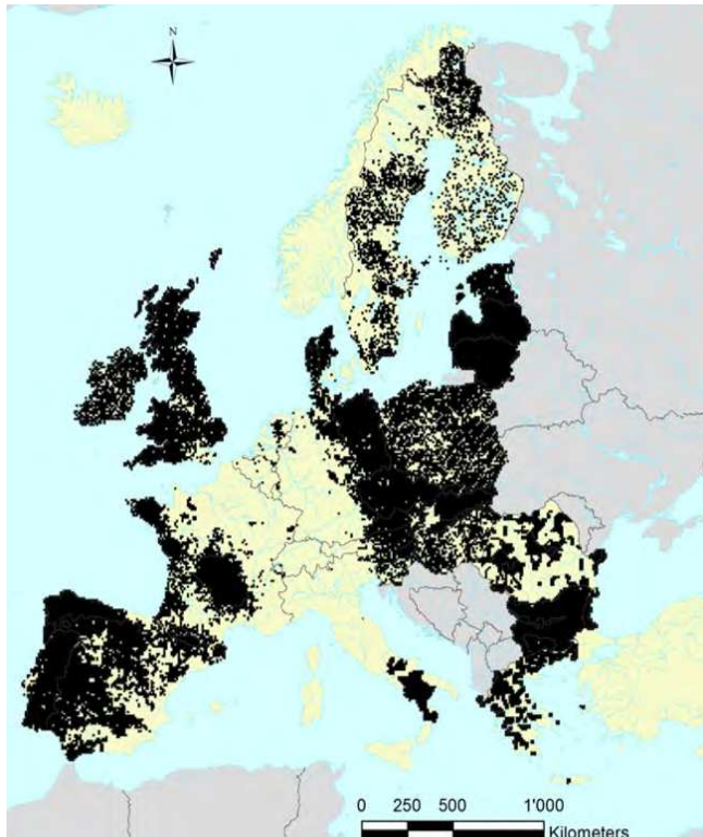
Figure 3 : Répartition de la Loutre d'Europe dans l'Union Européenne et quelques pays limitrophes (© Agence Européenne de l'Environnement, 2012).
