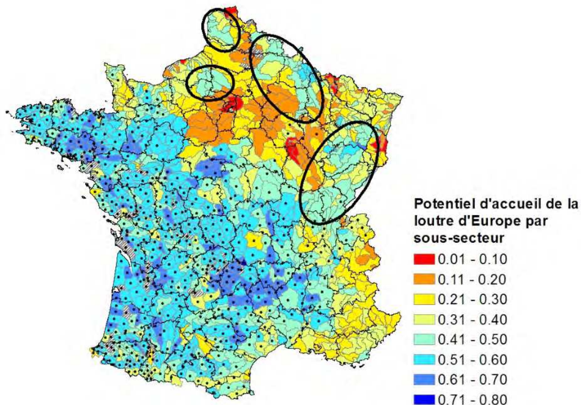
Figure 15 : Modèle du potentiel d'accueil de la Loutre d'Europe en France métropolitaine (© SPN/MNHN 2015)
