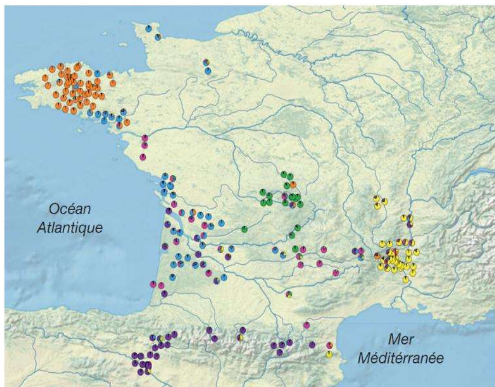
Figure 8 : Représentation géographique des six groupes génétiques mis en évidence (une couleur différente est assignée à chaque groupe génétique). Les diagrammes représentent pour chaque individu les probabilités d'appartenance à chacun des six groupes définis (Pigneur L.-P et al. 2018 – Apport de la génétique pour l'étude de la dynamique des populations de Loutre d'Europe Lutra lutra (L., 1758) en France. Naturae , 6 : 63-71.
